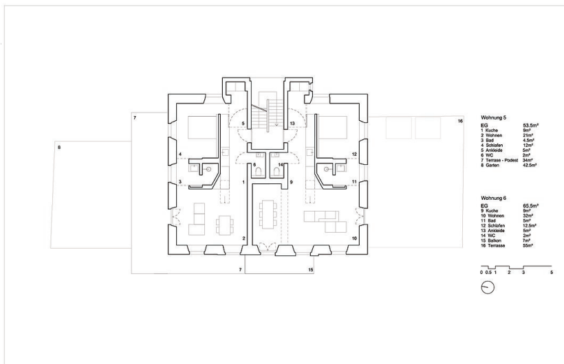
Grundriss WHG 5,6
