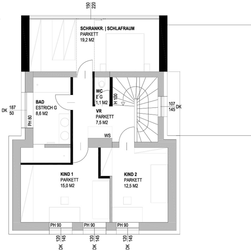
Grundriss OG
