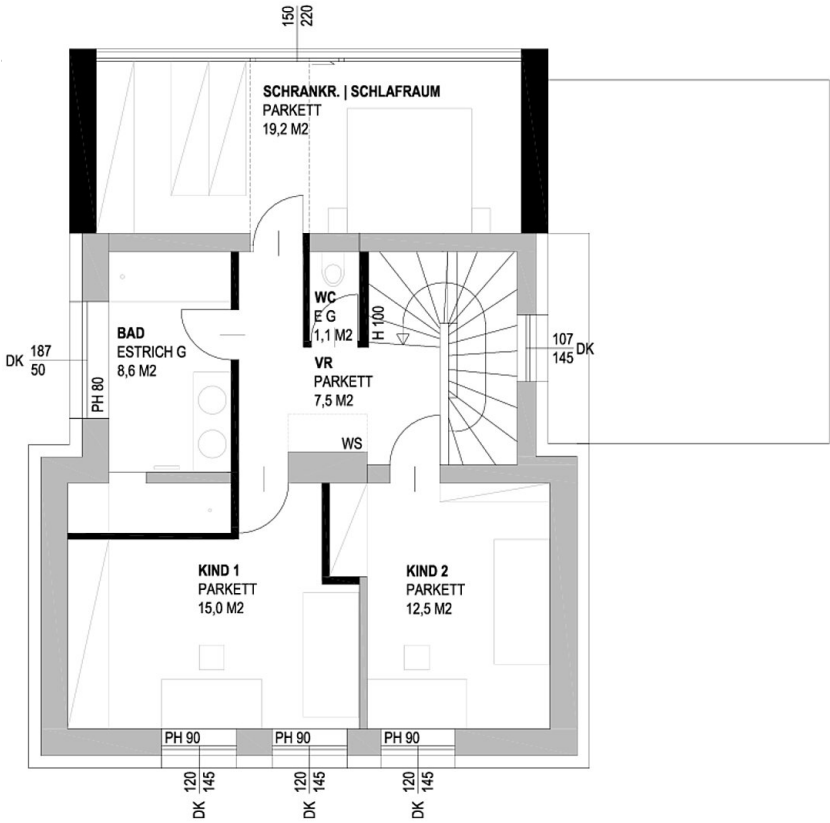
Grundriss OG
