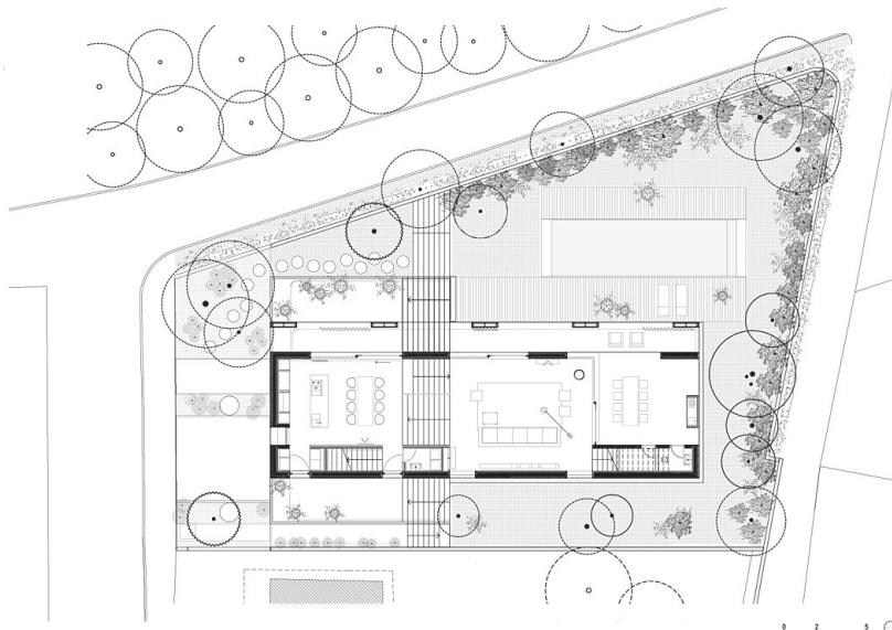
Grundriss EG2
