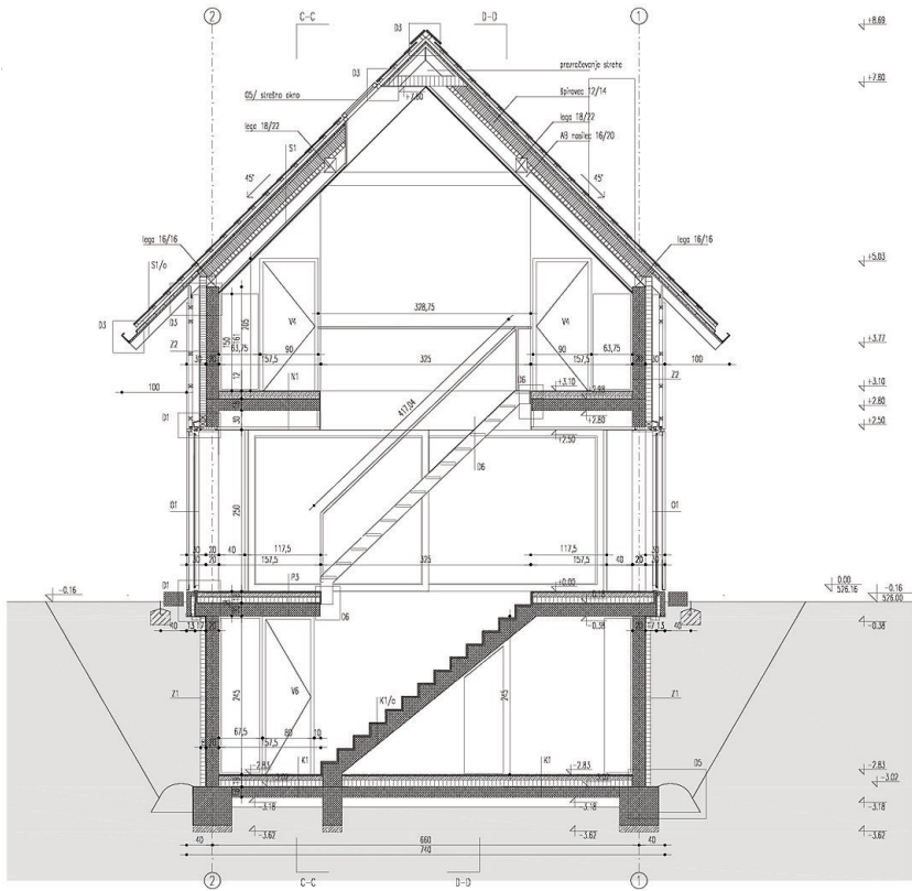
Schnitt
