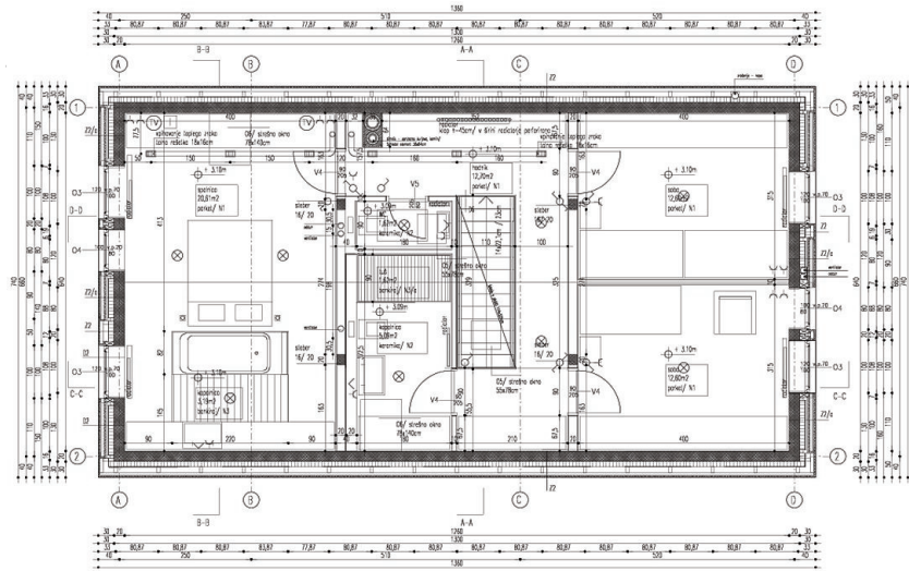
Grundriss OG
