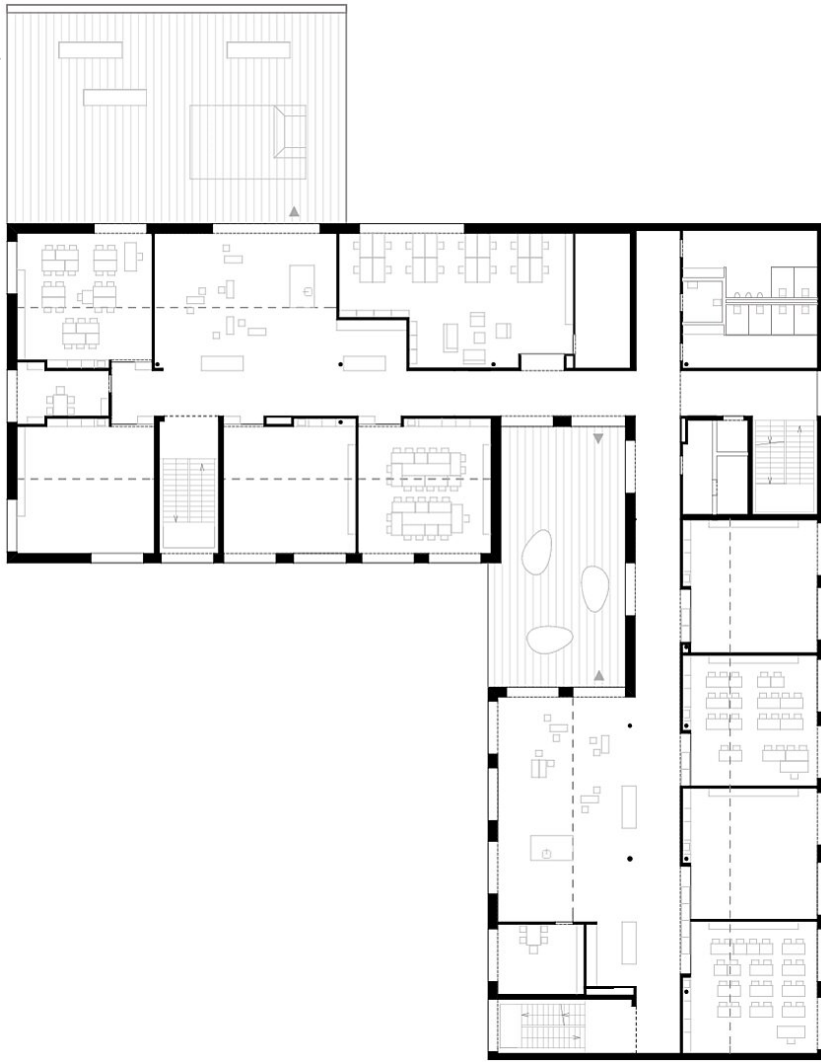
Grundriss OG2
