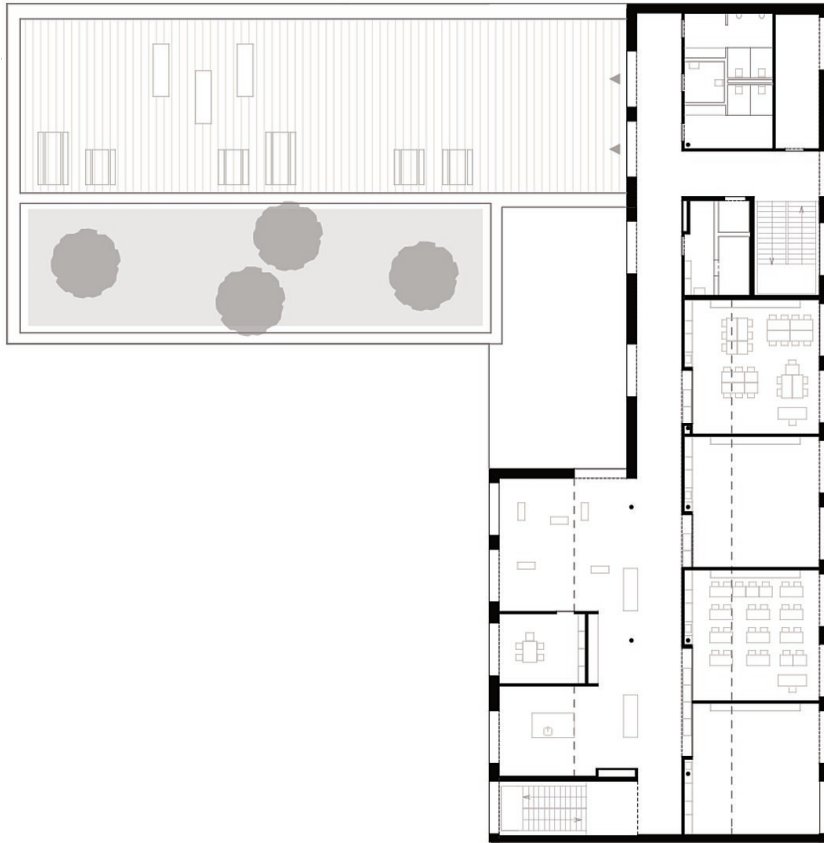
Grundriss OG3
