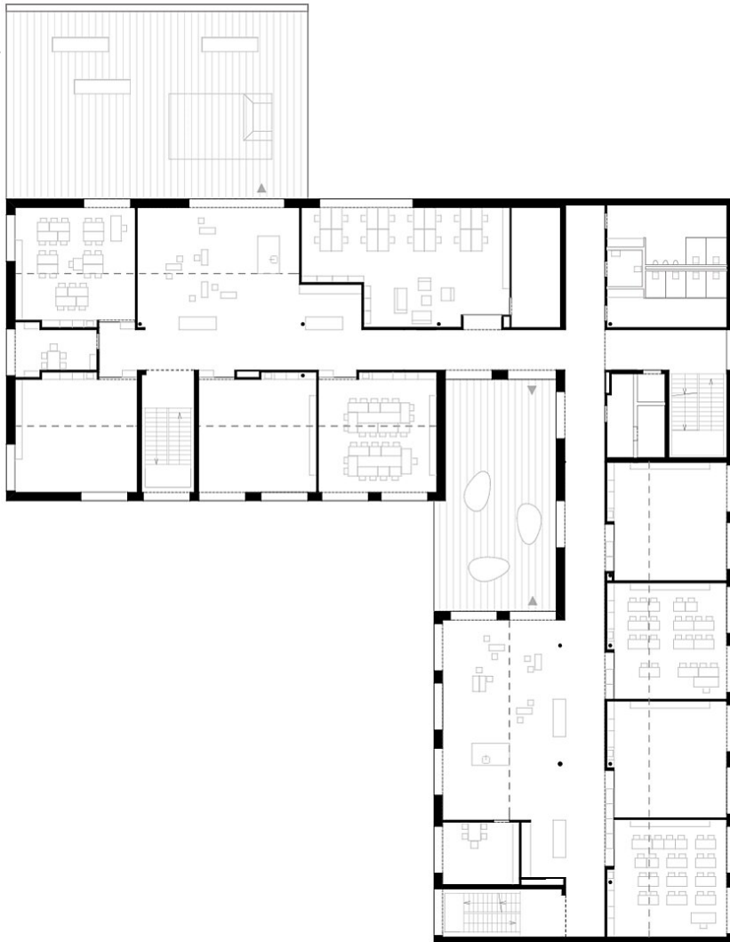
Grundriss OG2
