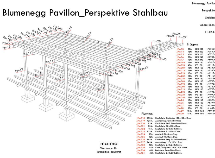
Perspektive Stahlbau
