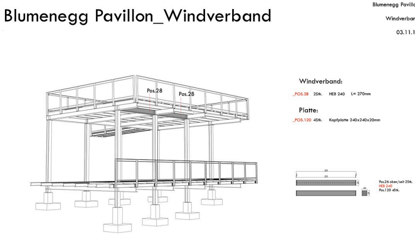
Perspektive Windverband
