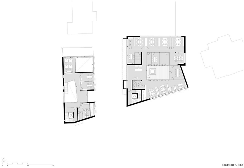
GRUNDRISS OG1 1:250
