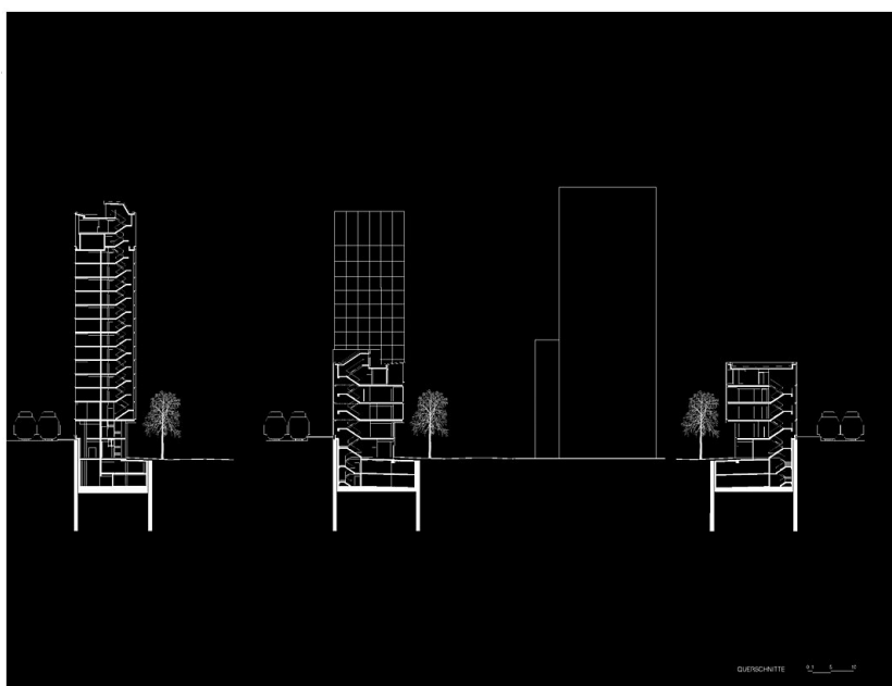
07 QUERSCHNITTE
