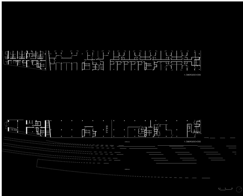
03 OBERGESCHOSS 01 04
