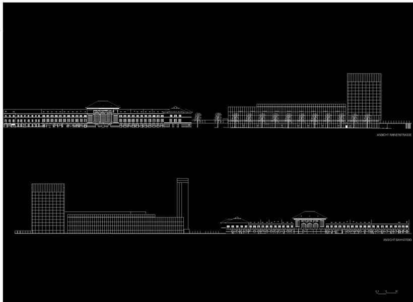
05 ANSICHTEN
