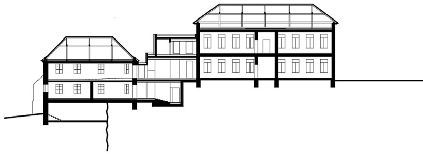
schnitt bb
