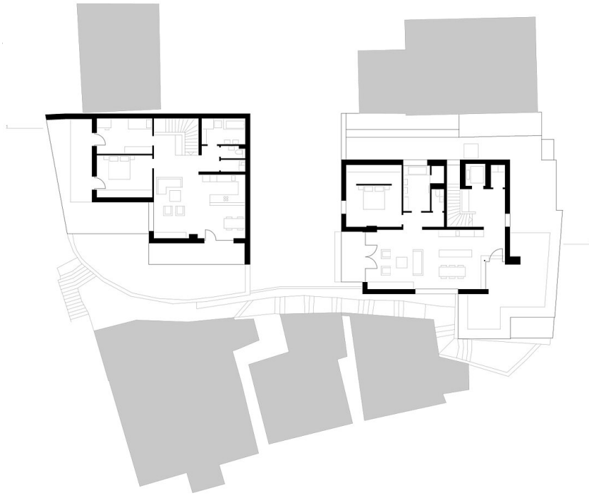
Grundriss OG3
