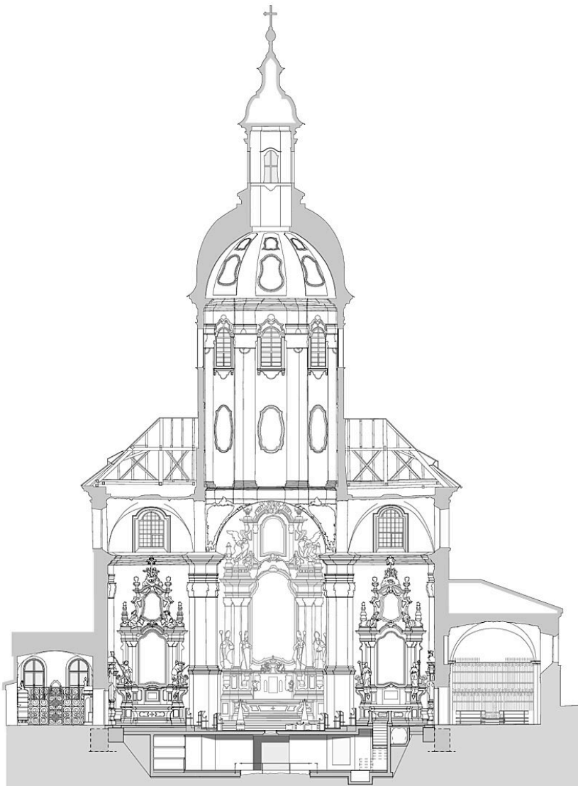
Querschnitt
