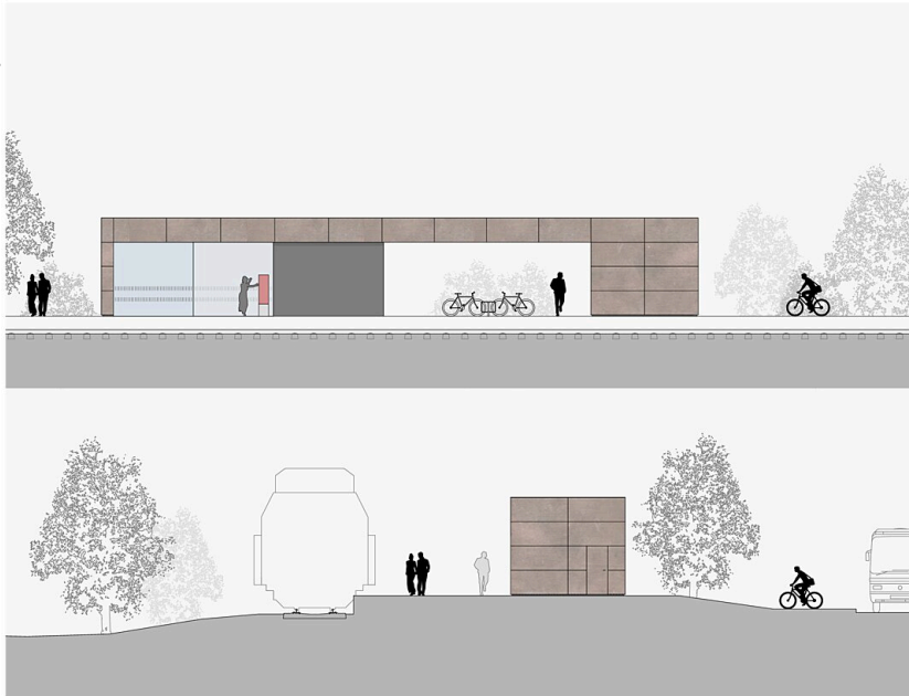
Ansichten 01
