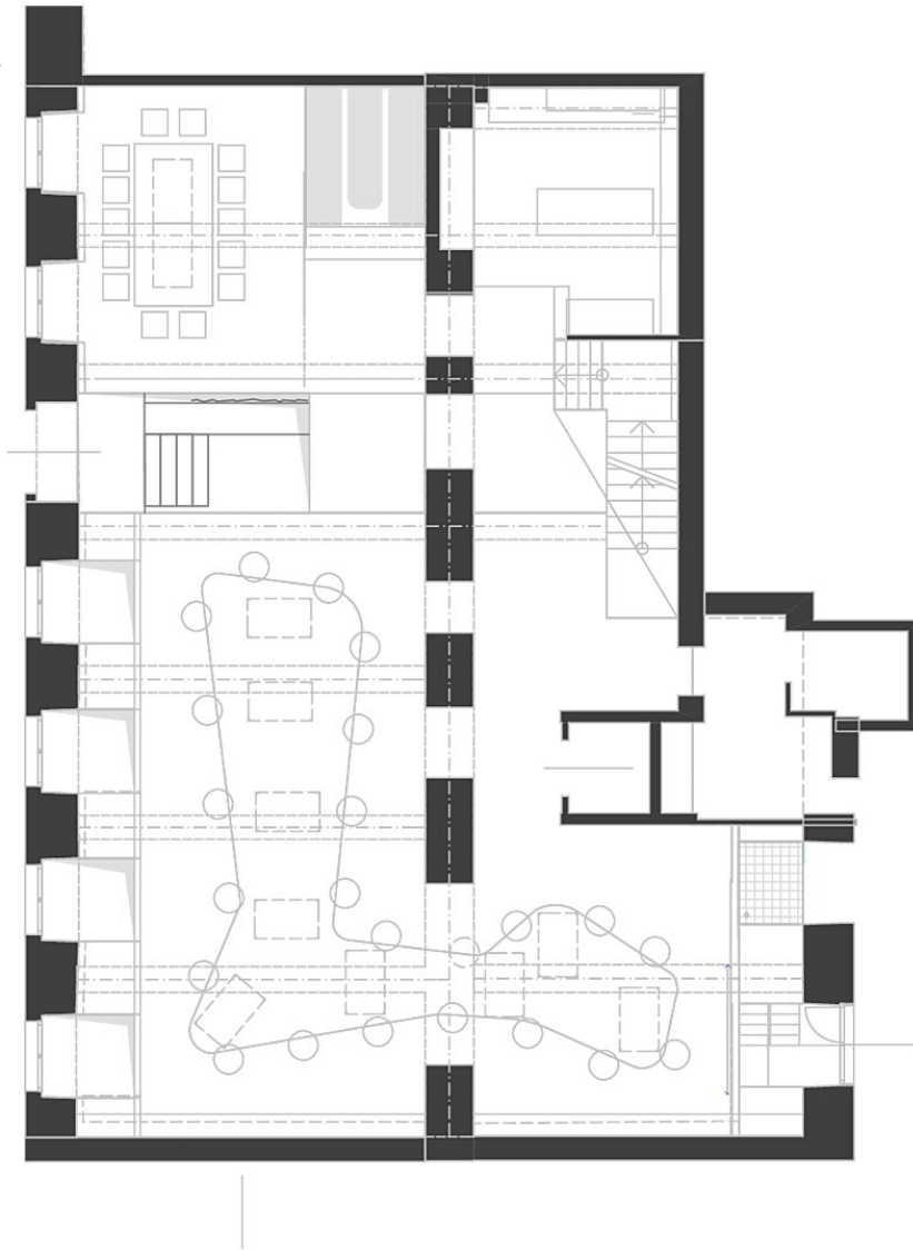
Grundriss OG
