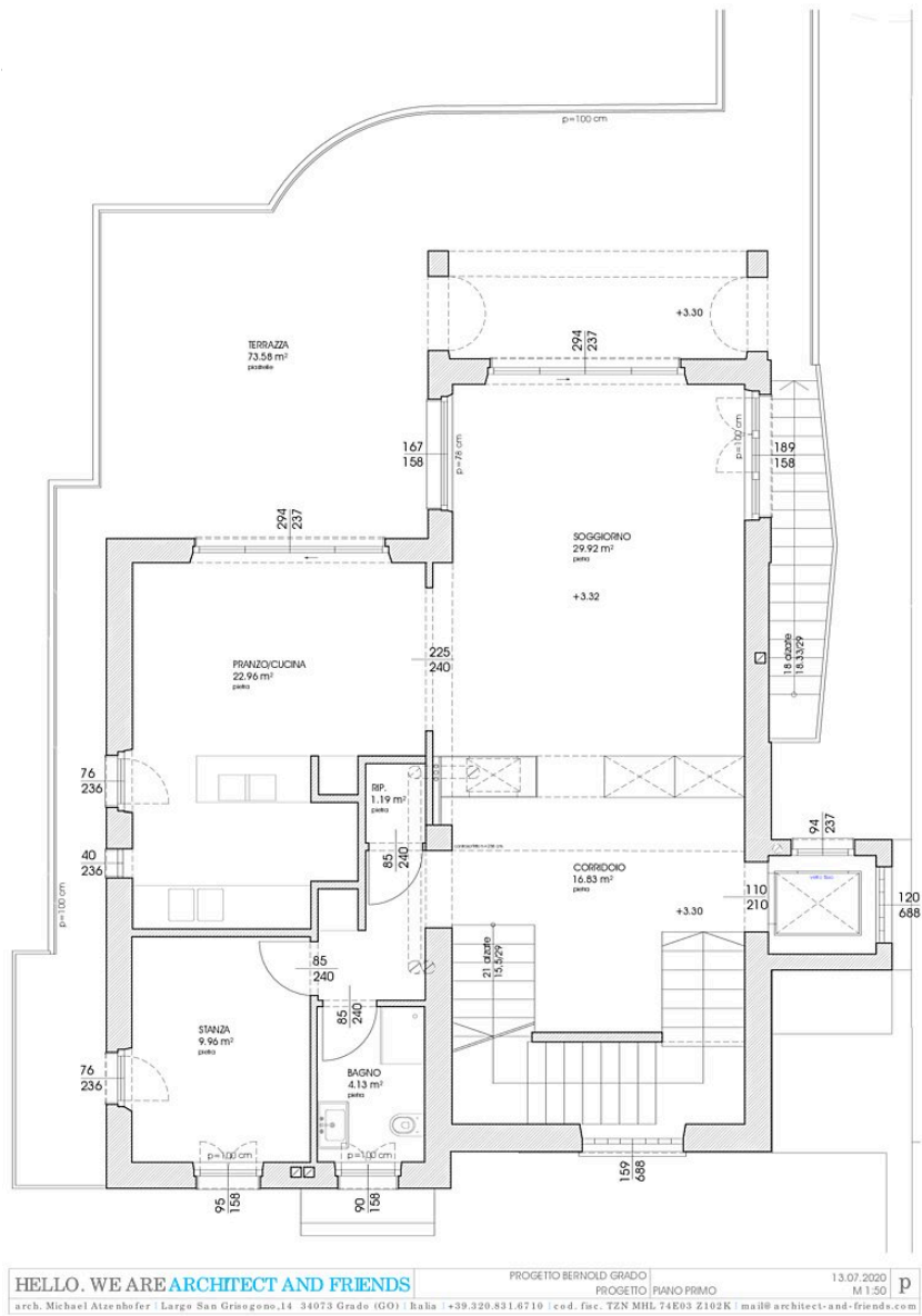
Grundriss OG1
