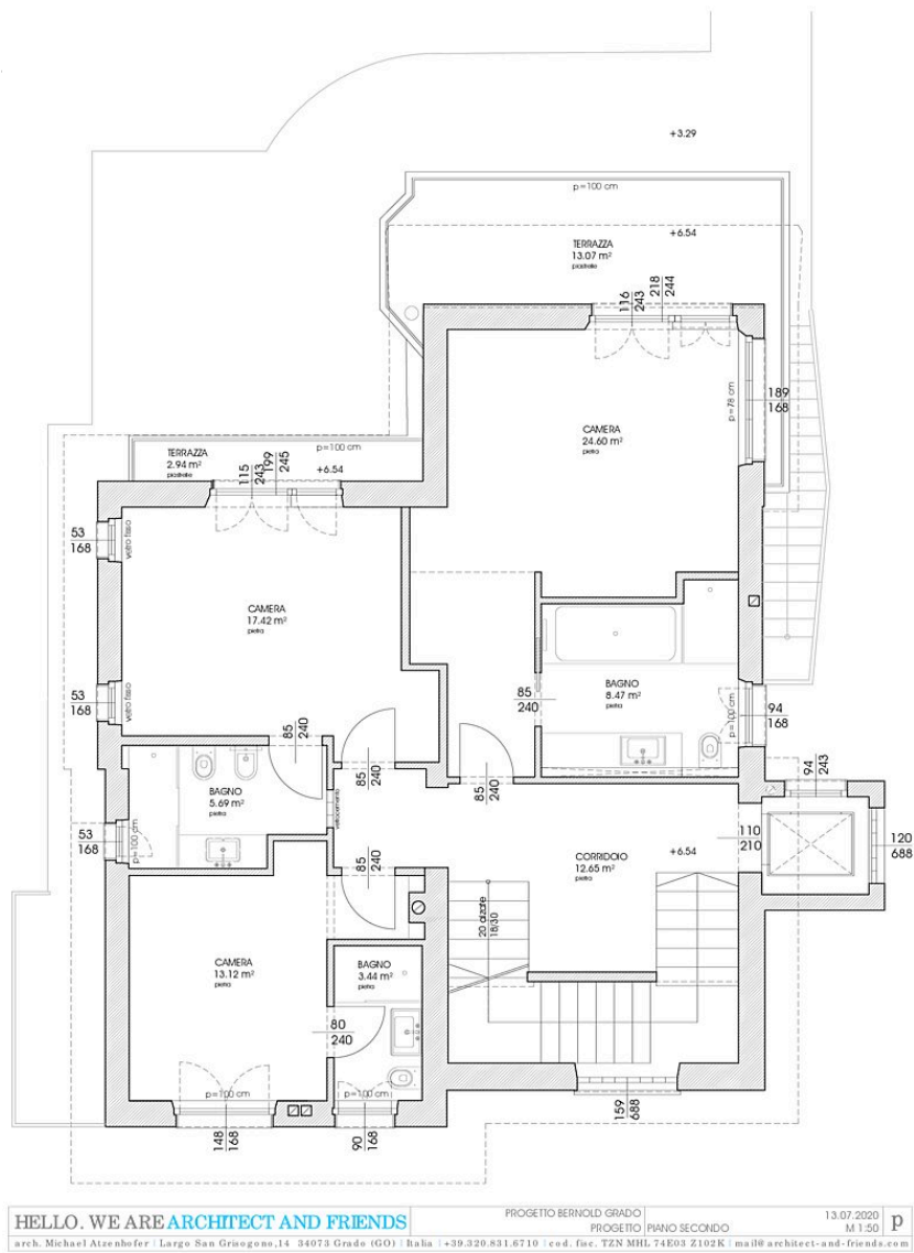
Grundriss OG2
