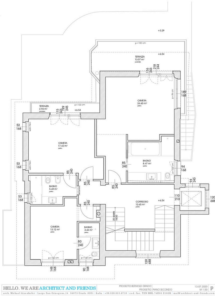
Grundriss OG2
