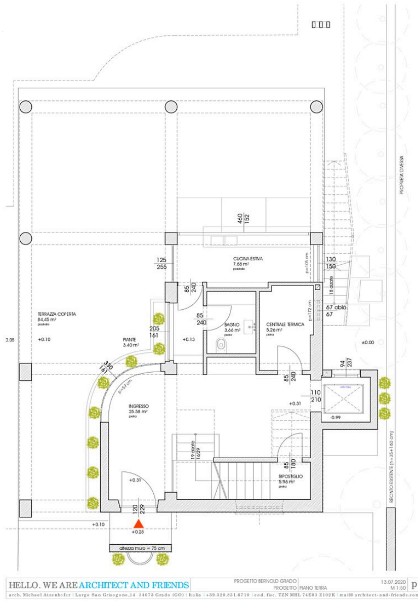
Grundriss EG
