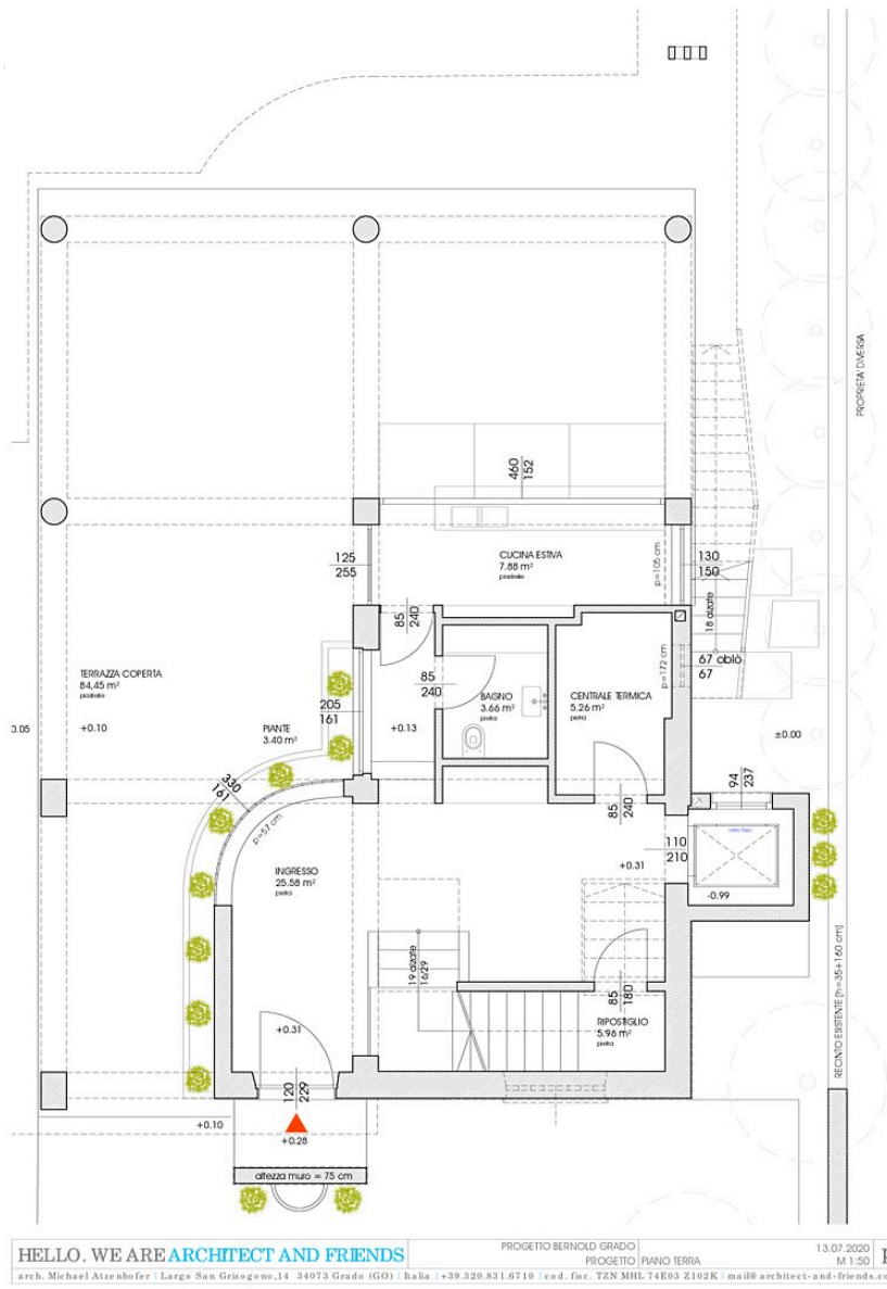
Grundriss EG
