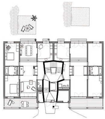
Wohnungstyp S-Haus EG
