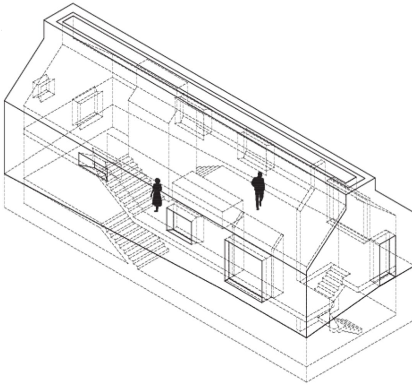
Axionometrie
