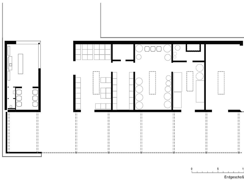
Grundriss EG
