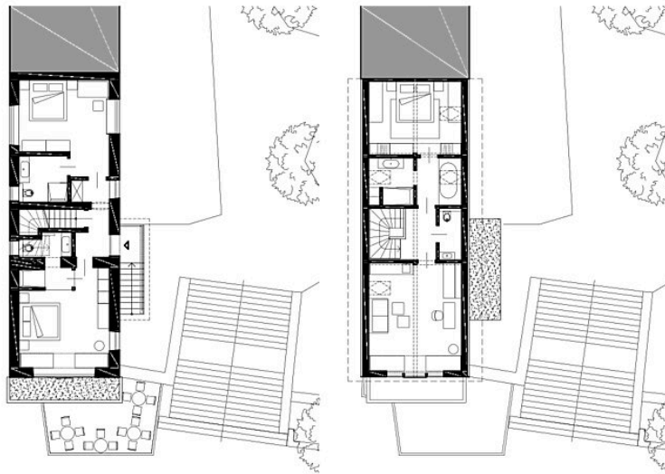
1. Obergeschoss 1/200
