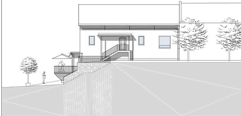
Ostansicht 1/200
