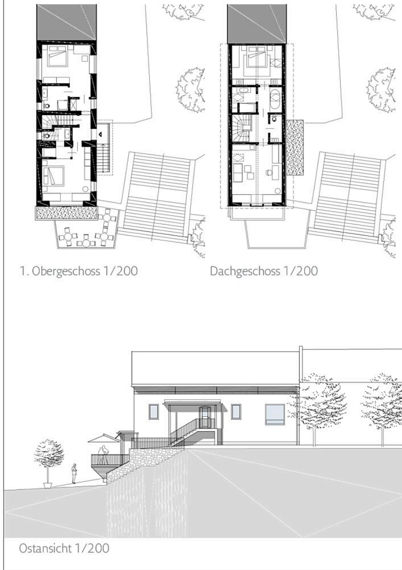
1642 DER KLEINE BÄR Grundrisse, Ansicht
