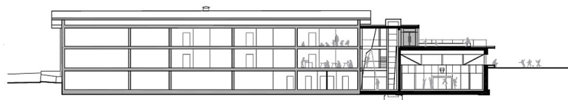
Schnitt C 1 5 10m
