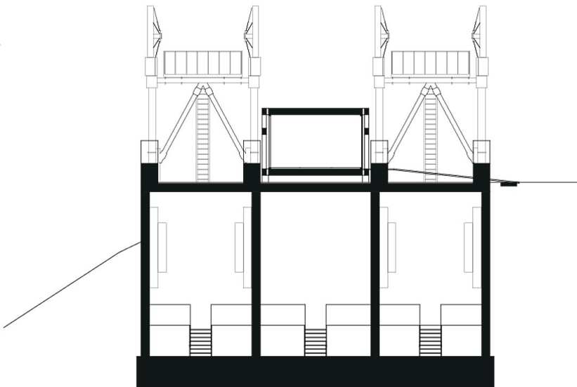
Querschnitt Bergstation
