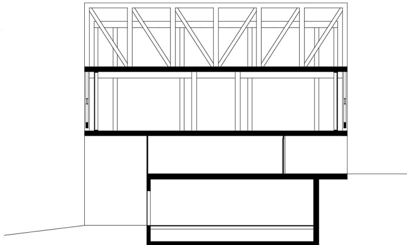
Querschnitt Talstation
