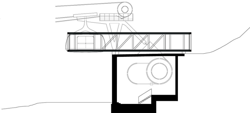
Längsschnitt Bergstation
