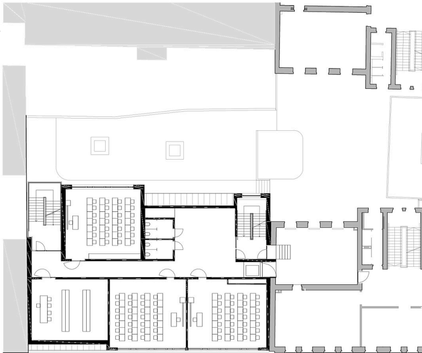
Grundriss DG
