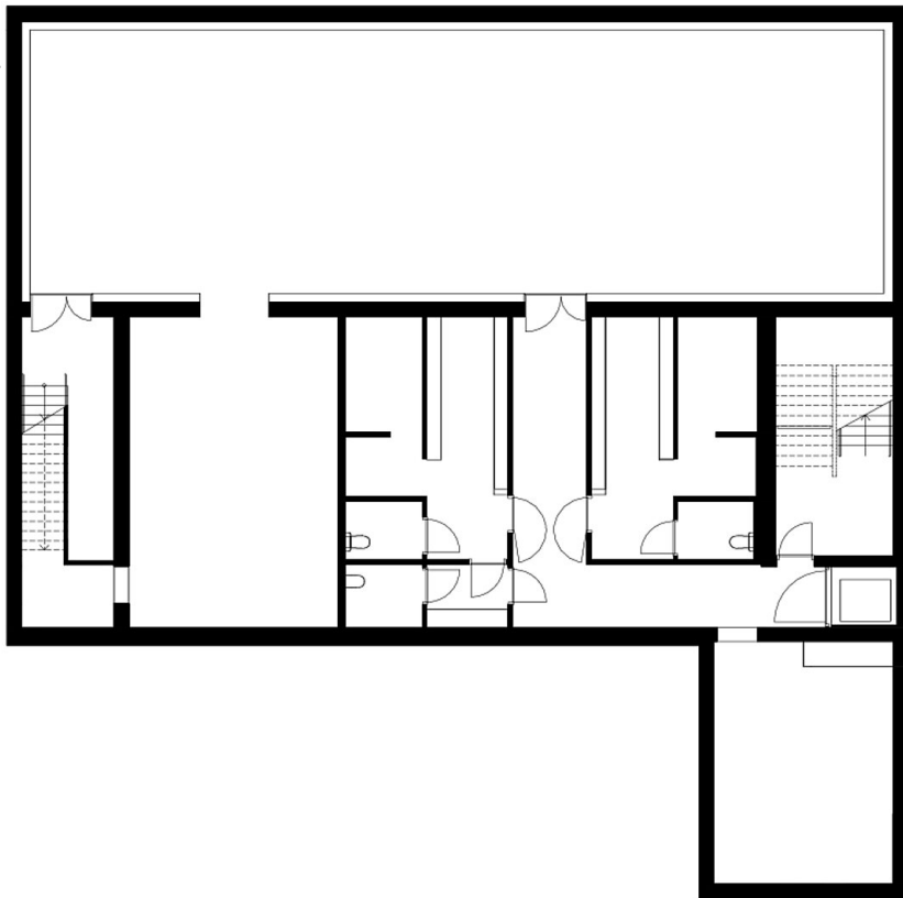
Grundriss UG2
