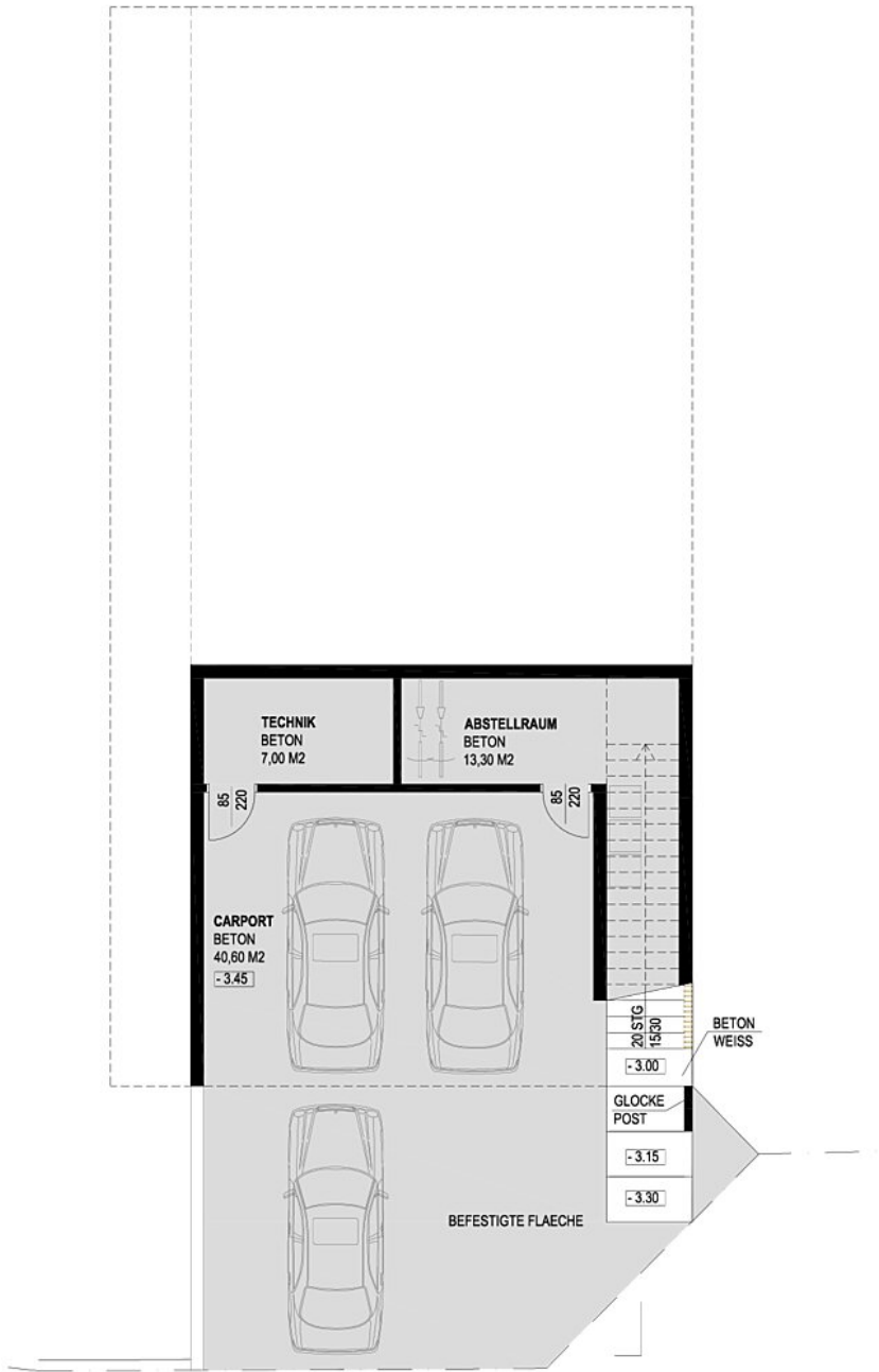
Grundriss EG
