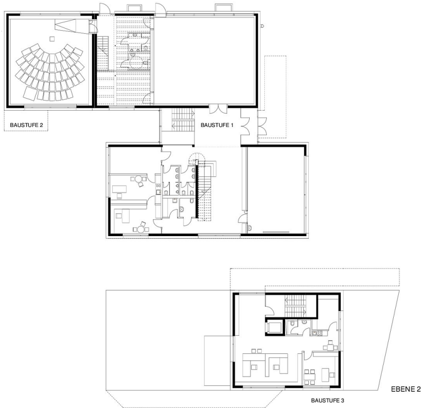
Grundriss Ebene 2
