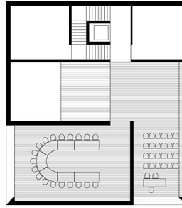
Grundriss OG2
