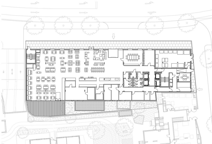
Erdgeschoss EG
