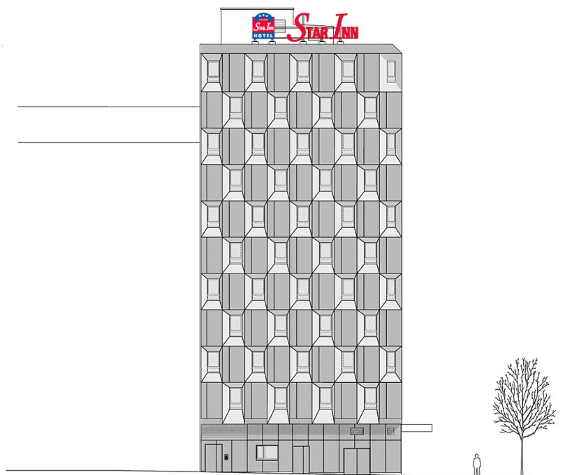
Ansicht Ost
