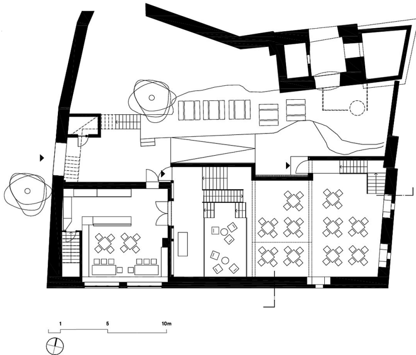
Eingangsebene
