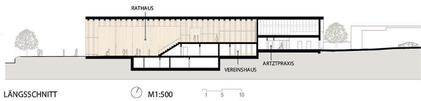
Längsschnitt
