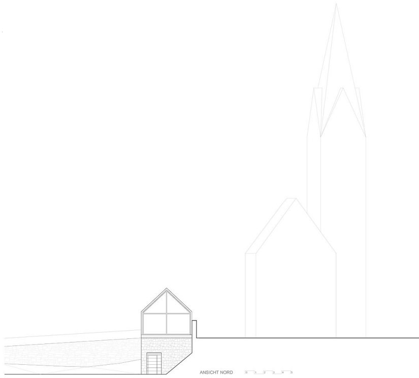
Ansicht Nord
