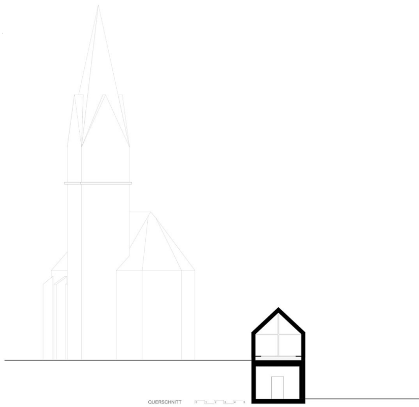
Querschnitt
