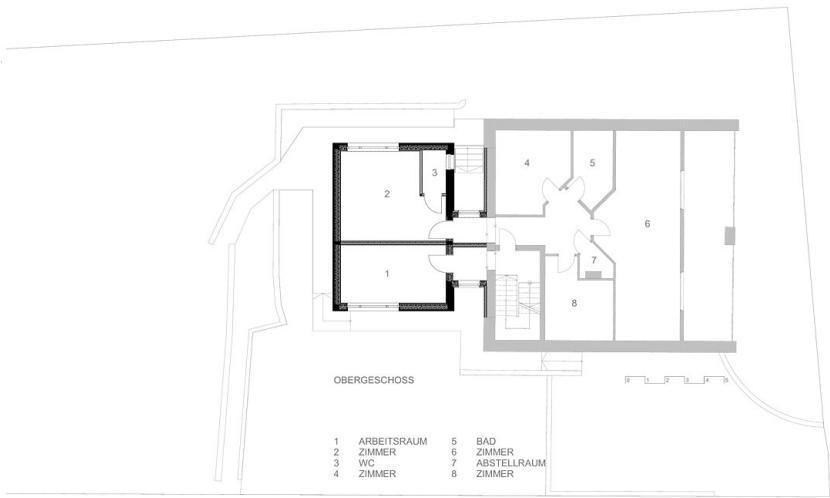
Grundriss OG
