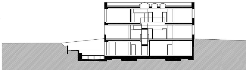
Schnitt B-B
