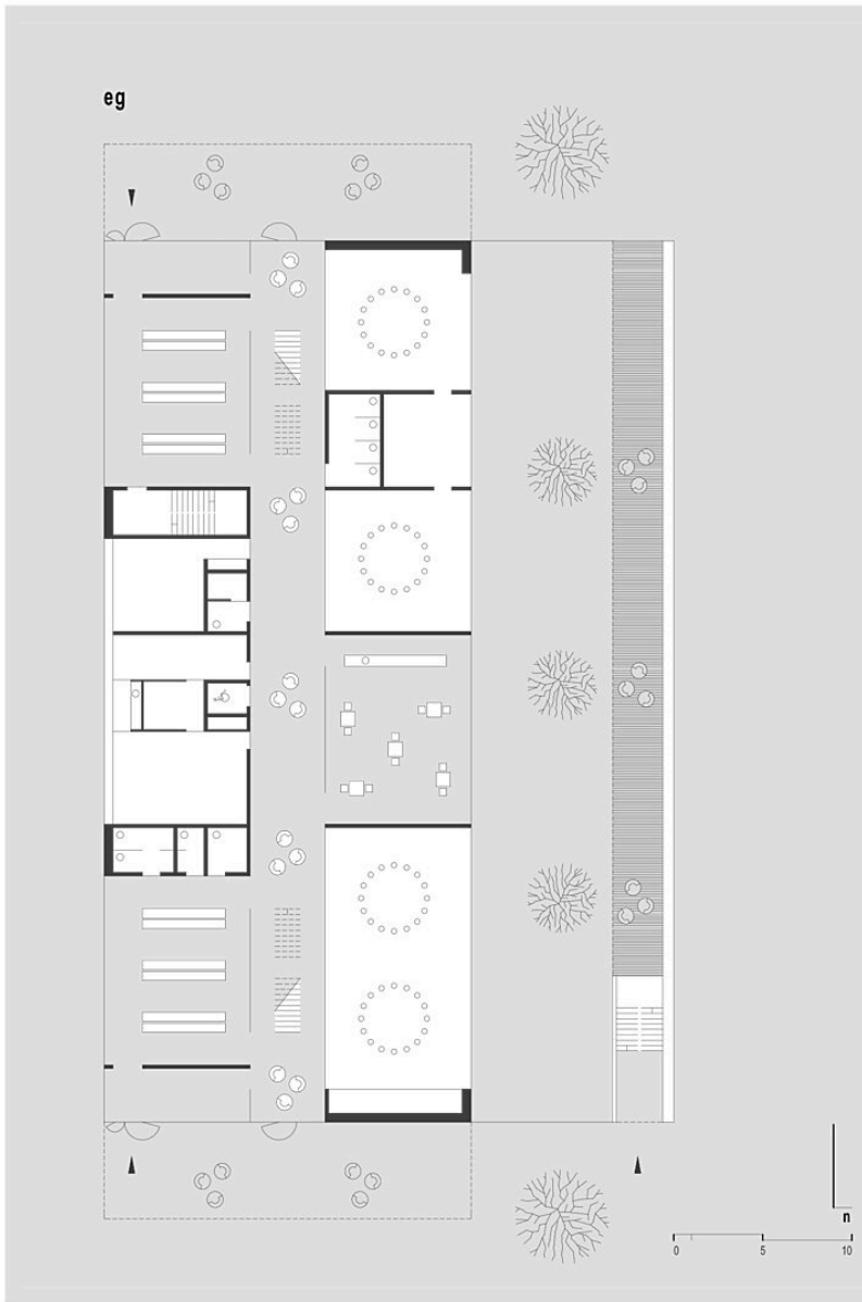
Grundriss EG
