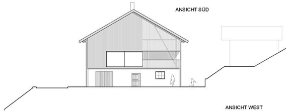
ANSICHT WEST ANSICHTEN M 1:200 10 5 1
