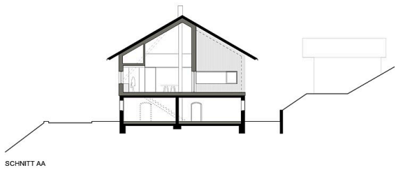
SCHNITT 10 5 1 M 1:200
