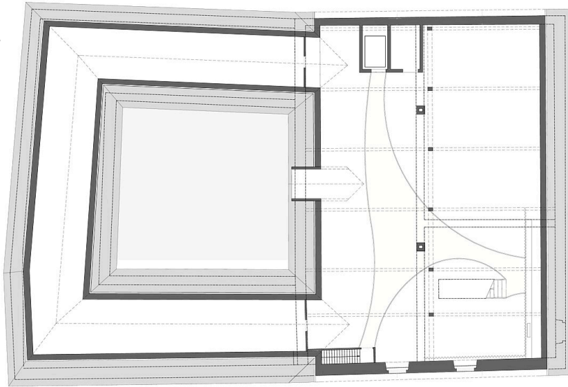
Grundriss DG1
