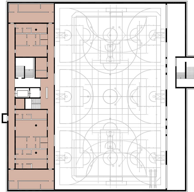
Grundriss UG3
