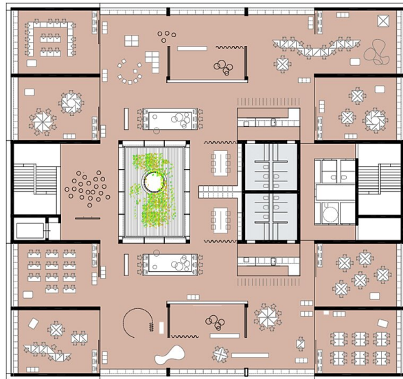
Grundriss OG2
