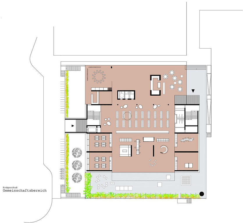
Grundriss EG
