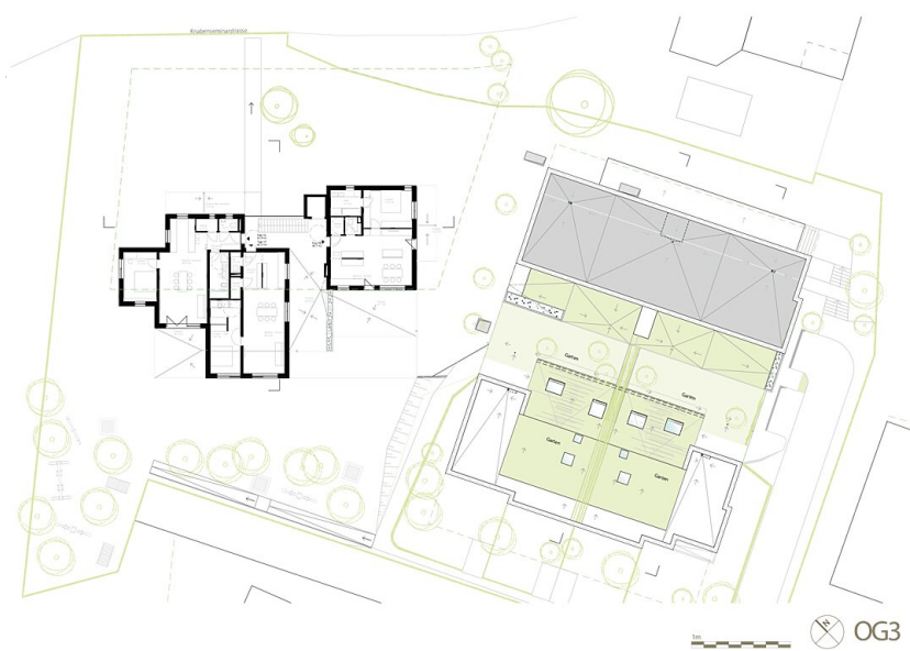
Grundriss OG3
