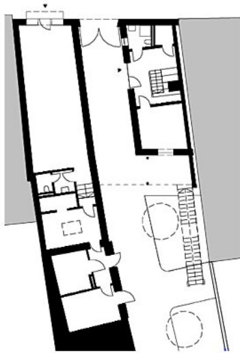
Grundriss EG
