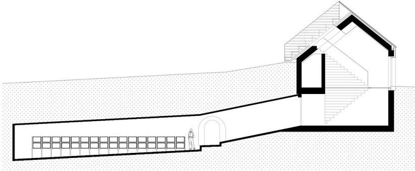
Grundriss, Schnitt
