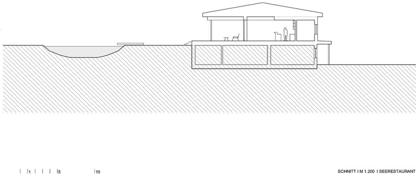
Schnitt
