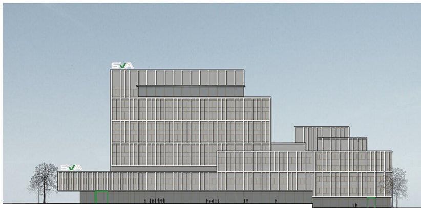
ANSICHT ZIEGELFENGASSE
