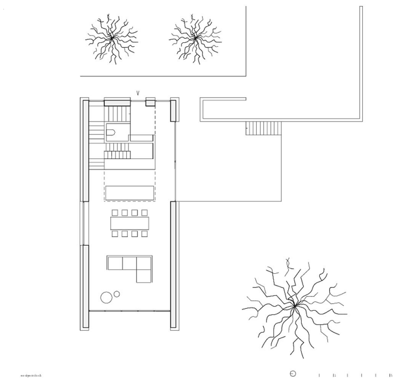
Grundriss EG
