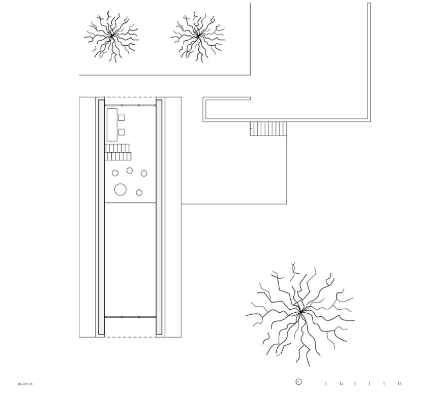
Grundriss Galerie
