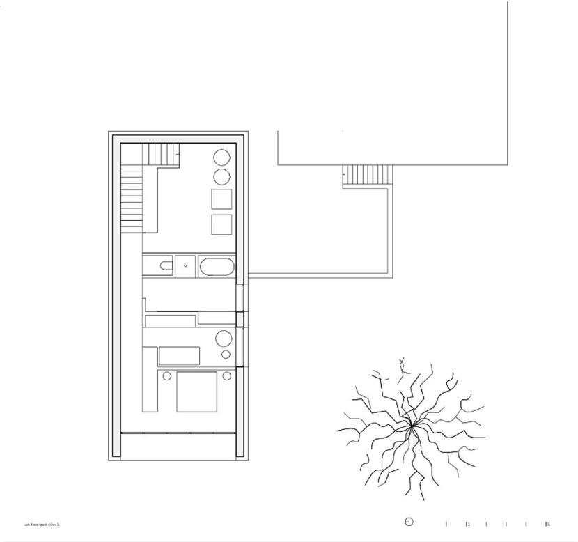
Grundriss UG
