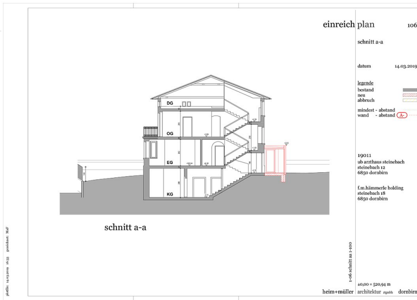
Schnitt AA
