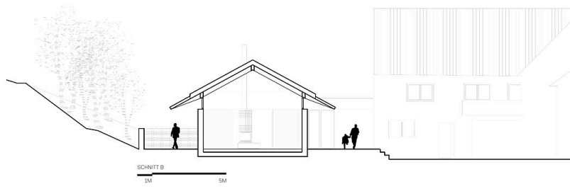
Schnitt B
