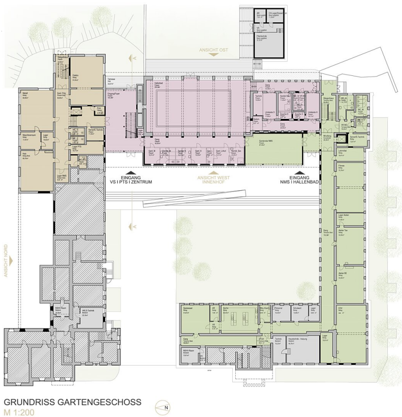
Grundriss Gartengeschoss
