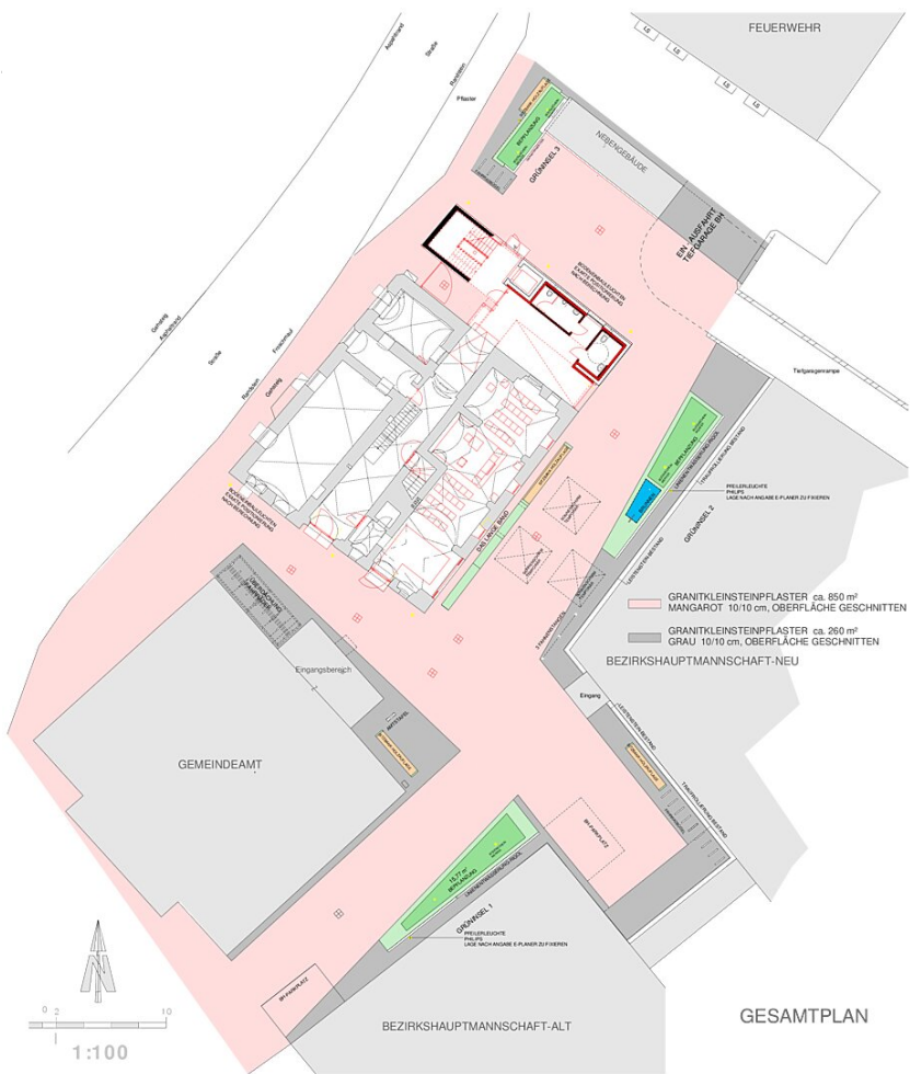
Gesamtplan
