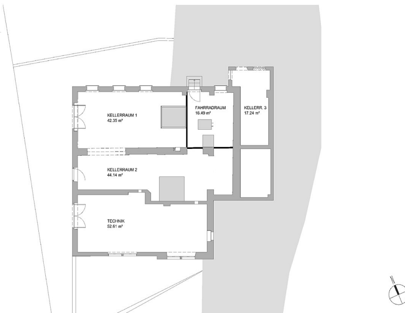
Grundriss KG
