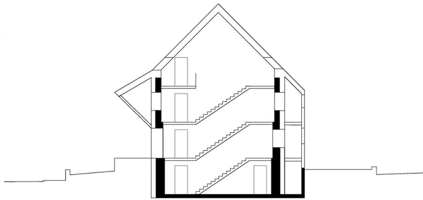
SCHNITT AA 0 5
