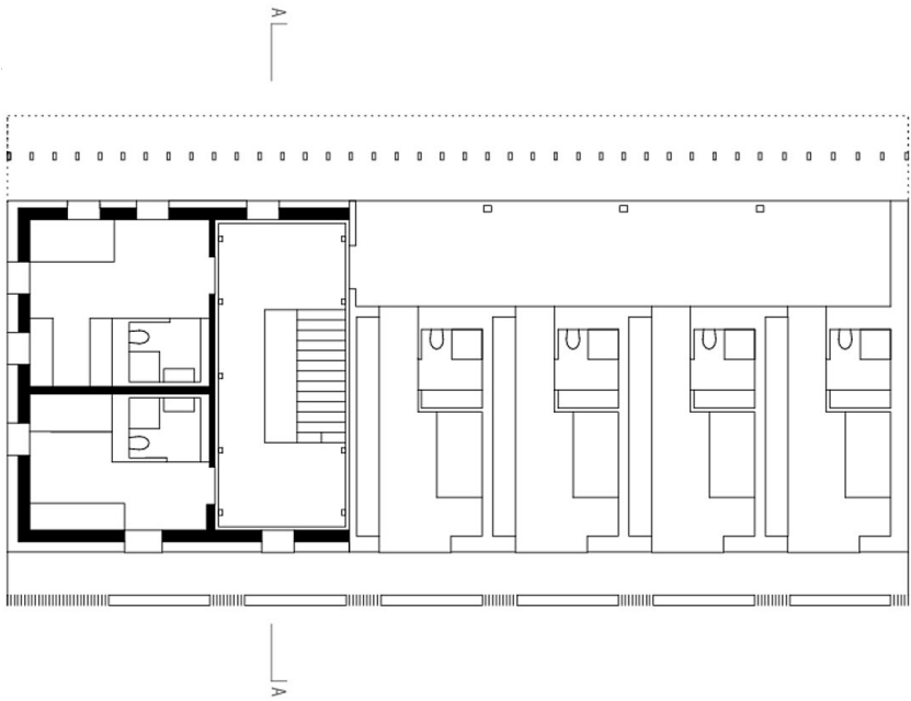
0BERGESCHOSS
