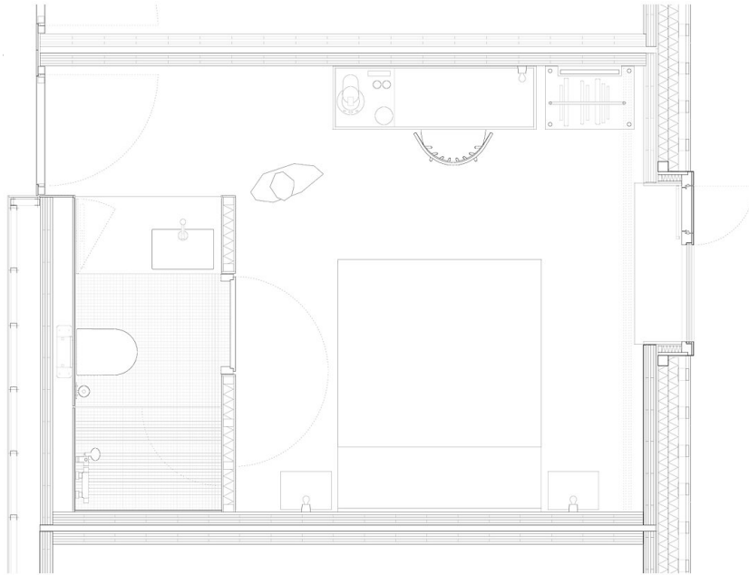
Grundriss Zimmer
