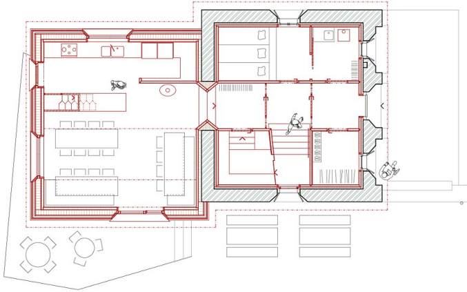
Grundriss EG
