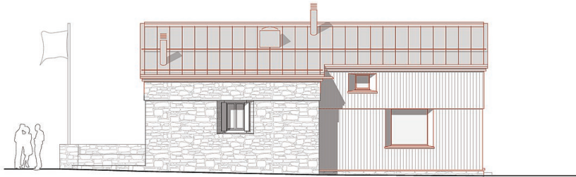
Ansicht Nord
